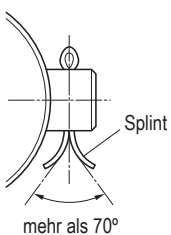
Biegeweise des Splints
