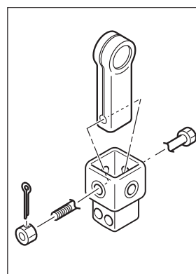
(Rollfahrwerk)
