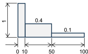
% Betriebszeit Lastspektrum 1
