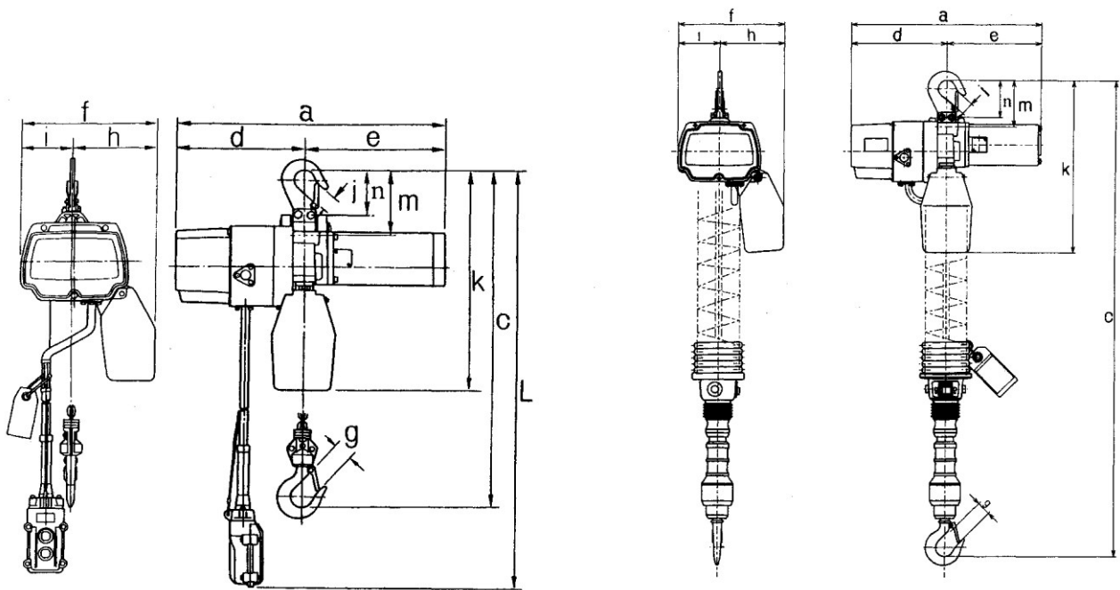
Ausführung mit und ohne Feinhub
