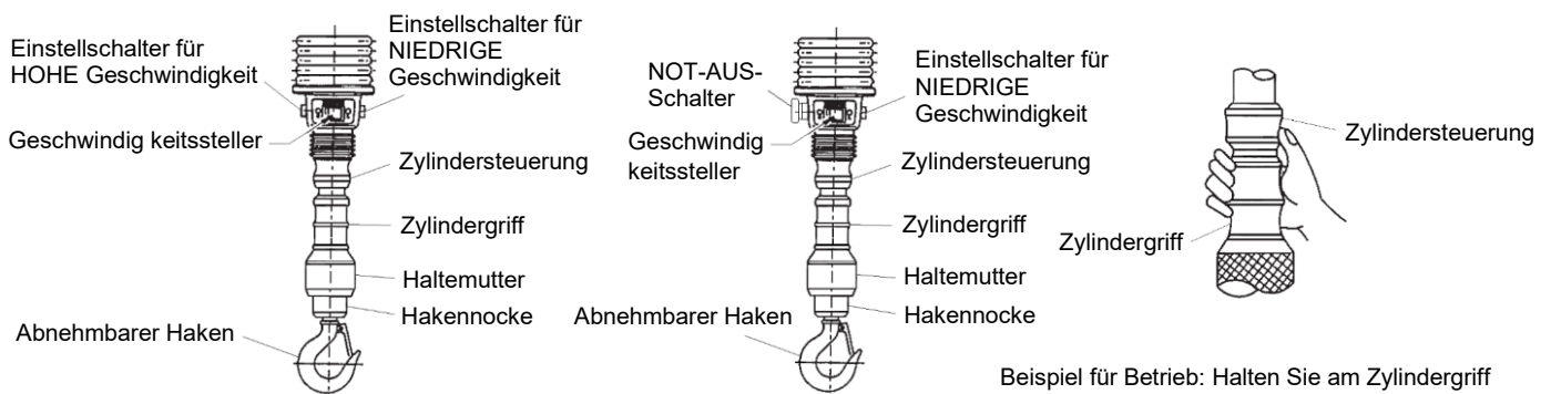
Ausführung mit NOT-AUS-Schalter
