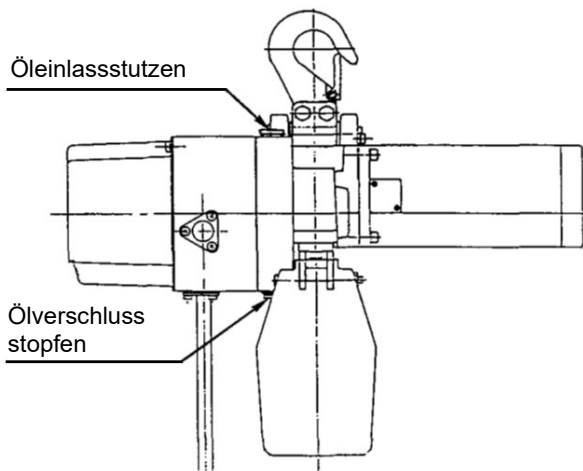
Verlangte Getriebeölmenge je nach Tragfähigkeit
