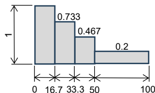
% Betriebszeit Lastspektrum 2
